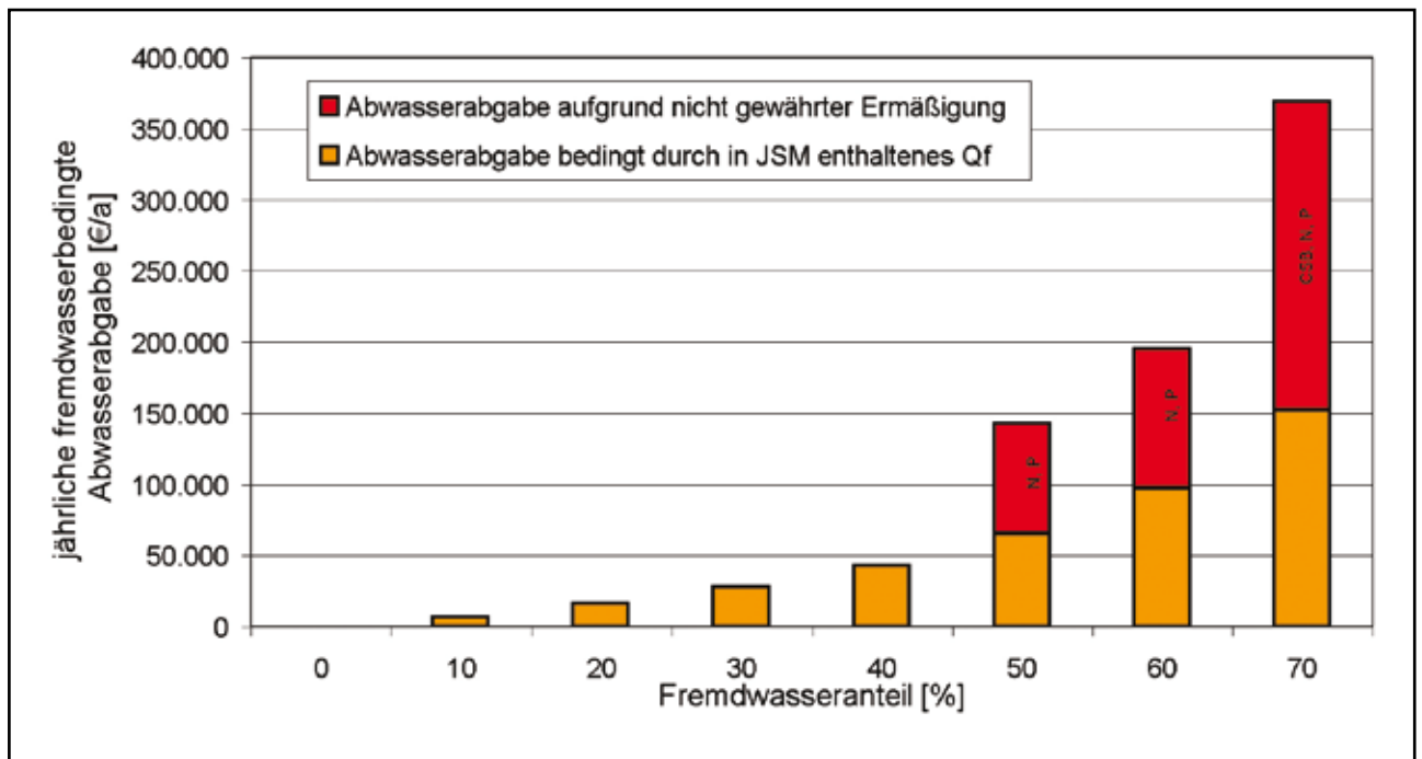
Abb. 20: Fremdwasserbedingte Abwasserabgabe für verschiedene FWA einer KA für 40.000 EW
