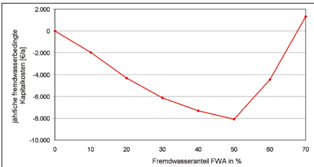
Abb. 17: Jährliche fremdwasserbedingte Kapitalkosten (Bau und Maschinentchnik) für Vorklärbecken, Belebungsbecken und Nachklärbecken bei verschiedenen Fremdwasseranteilen für eine Beispielanlage mit 40.000 EW
