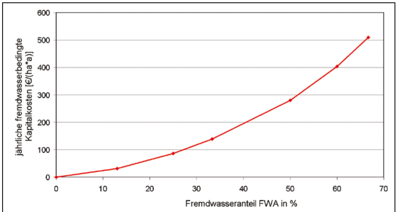
Abb. 15: Jährliche fremdwasserbedingte Kapitalkosten (Bau und Maschinentchnik) für ein typisches Regenüberlaufbecken bei verschiedenen Fremdwasseranteilen (Beispiel aus Abb. 14)
