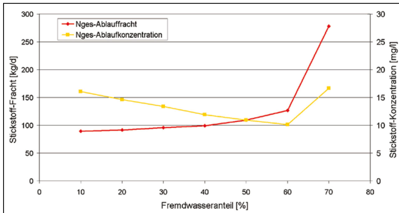
Abb. 10: N_{ges} -Ablaufmengen und -konzentrationen bei unterschiedlichen Fremdwasseranteilen
