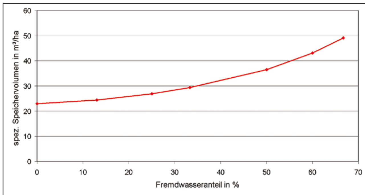
Abb. 14: Spezifisches Speichervolumen eines fiktiven Zentralbeckens bei unterschiedlichen Fremdwasseranteilen nach Decker (1998)
