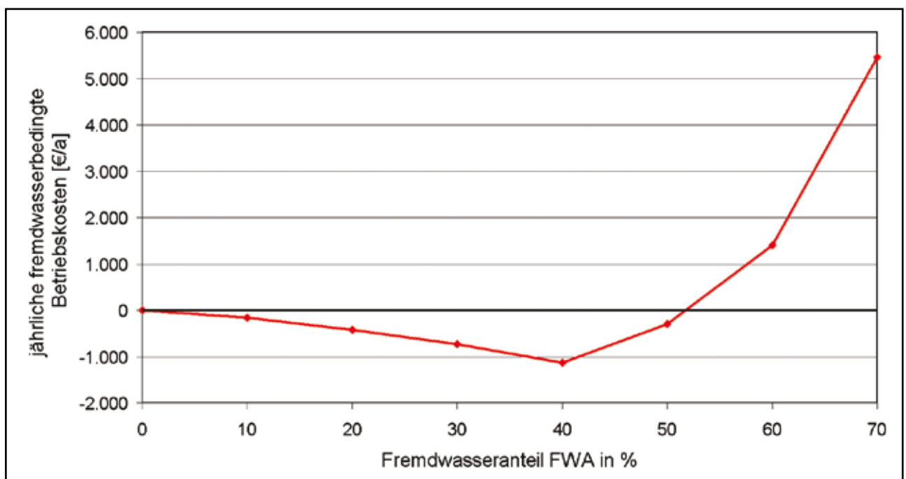
Abb. 18: Jährliche fremdwasserbedingte Betriebskosten bei verschiedenen Fremdwasseranteilen für eine Beispielanlage mit 40.000 EW
