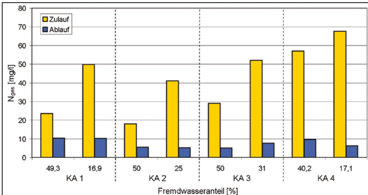
Abb. 12: Durchschnittliche N_{ges} Zu- und Ablaufkonzentrationen bei hohen und niedrigen Fremdwasseranteilen für vier Kläranlagen. Linke Balkenpaare jeweils Werte von September 2002, rechte Balkenpaare Werte von September 2003
