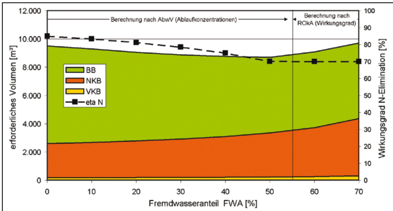
Abb. 16: Erforderliche Volumina für Vorklärbecken, Belebungsbecken und Nachklärbecken sowie Wirkungsgrad der Stickstoffelimination bei Fremdwasseranteilen zwischen 0 und 70 %
