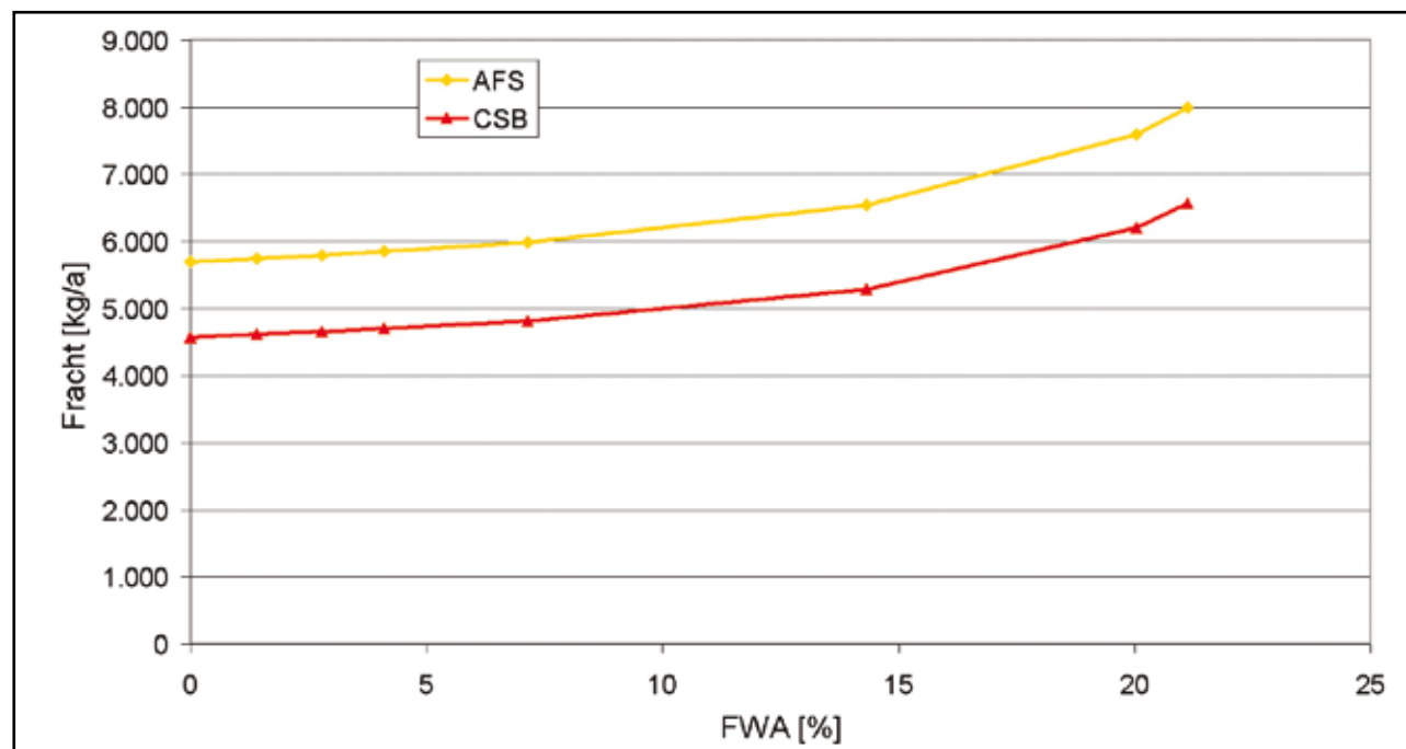
Abb. 9: Entlastete AFS- und CSB-Frachten eines Regenüberlaufbeckens im Hauptschluss bei unterschiedlichen Fremdwasseranteilen
