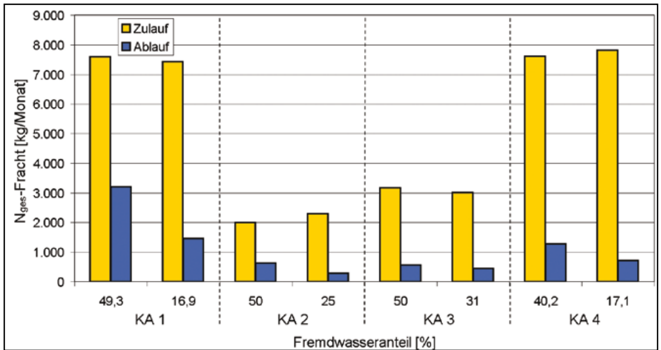
Abb. 13: N_{ges} Zu- und Abflafrachten bei hohen und niedrigen Fremdwasseranteilen für vier Kläranlagen. Linke Balkenpaare jeweils Werte von September 2002, rechte Balkenpaare Werte von September 2003
