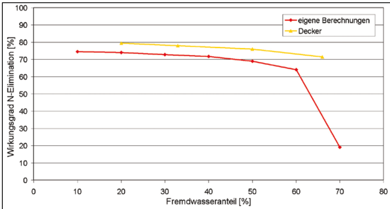
Abb. 11: Wirkungsgrad der Stickstoffelimination bei verschiedenen Fremdwasseranteilen, ergänzt um Werte nach Decker (1998)
