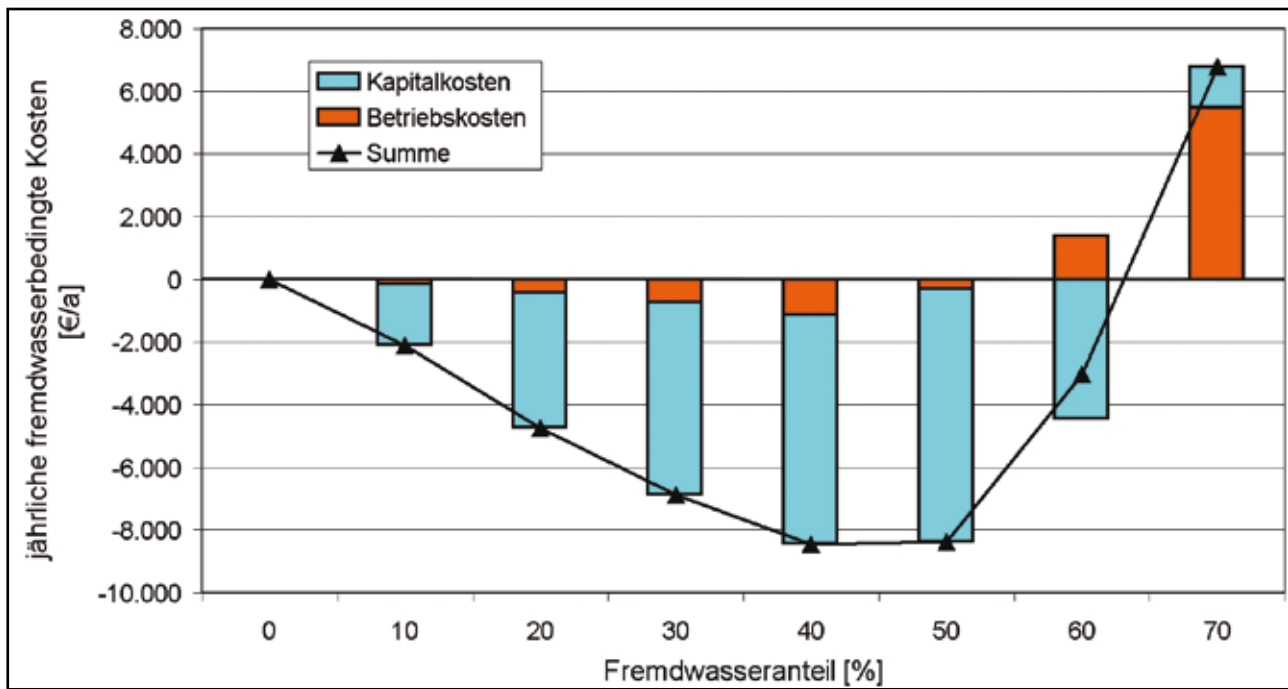
Abb. 19: Fremdwasserbedingte Jahreskosten für eine Beispielanlage mit 40.000 EW bei verschiedenen Fremdwasseranteilen
