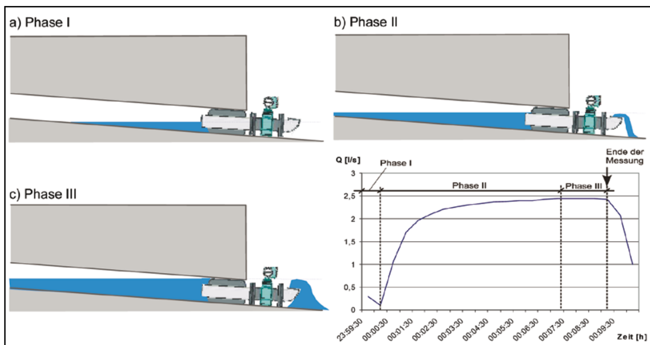
Abb. 17: Verlauf einer mobilen MID-Messung in drei Phasen (rechts unten): (a) Einstauphase, (b) Anstiegsphase, (c) Messphase
