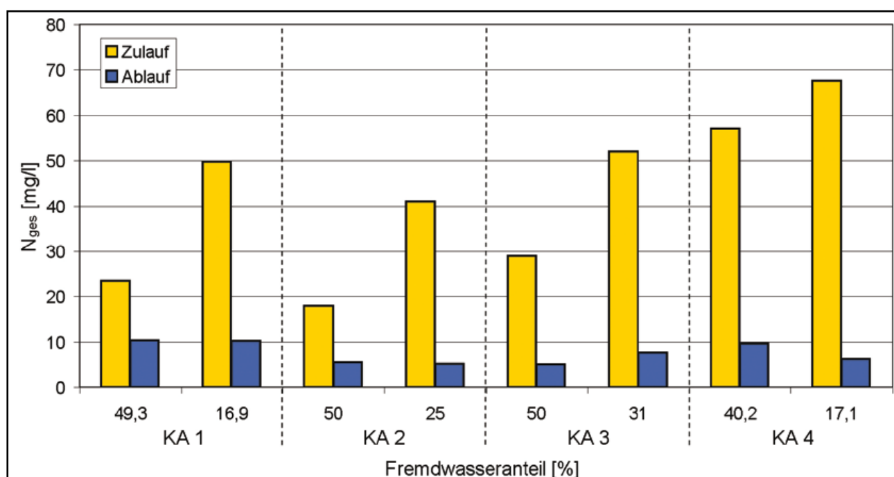
Abb. 34: Durchschnittliche N_{ges} Zu- und Ablaufkonzentrationen bei hohen und niedrigen Fremdwasseranteilen für vier Kläranlagen. Linke Balkenpaare jeweils Werte von September 2002, rechte Balkenpaare Werte von September 2003
