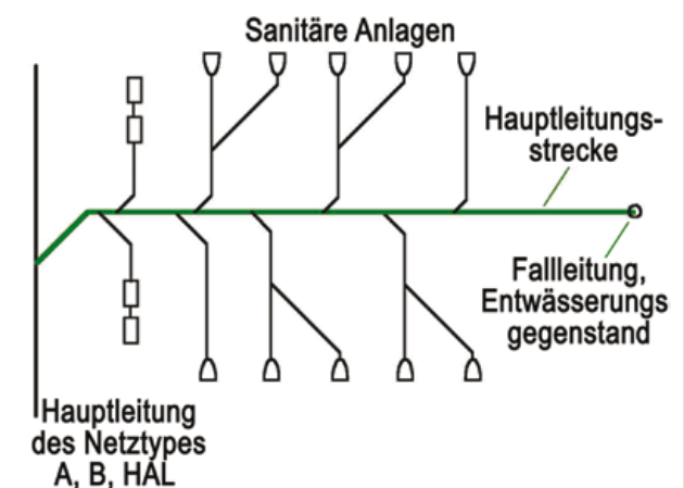
Abb. 53: Unterscheidung von Netztypen nach Zugänglichkeit und Komplexität der Entwässerungssysteme (Bosseler et al., 2003a)
