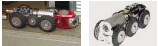
Abb. 56: Fahrwagen mit Schwenkkopfkamera (links) und Axialkopfkamera (rechts)
