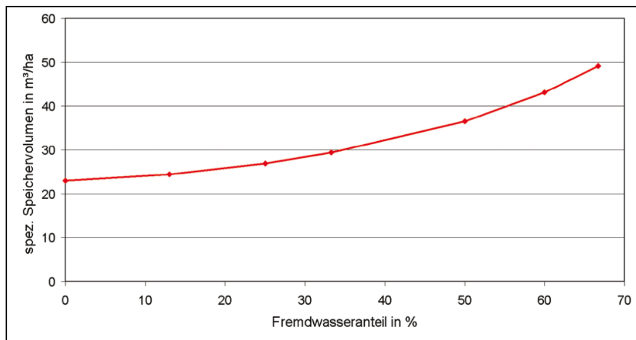
Abb. 39: Spezifisches Speichervolumen eines fiktiven Zentralbeckens bei unterschiedlichen Fremdwasseranteilen nach Decker (1998)
