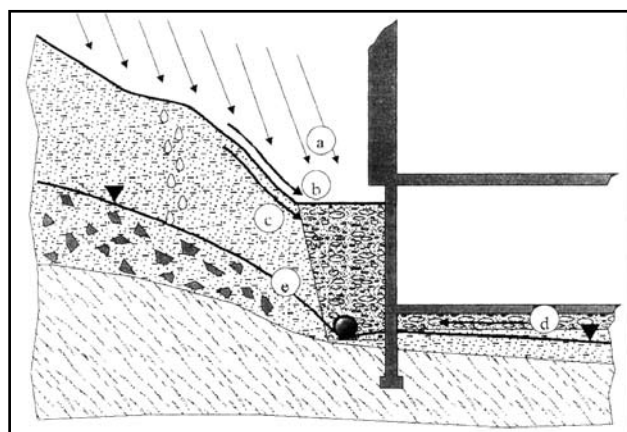
Abb. 79: Zuflüsse zu einer Hausdrainage in Hanglage: (a) direkte Präzipitation auf die Drainage, (b) Oberflächenzufluss, (c) hypodermischer Zufluss (Schichtenwasser), (d) Zuflüsse über gut wasserwegsame Horizonte, (e) Grundwasserzufluss aus dem Hangschuttbereich (Stein et al., 1995)
