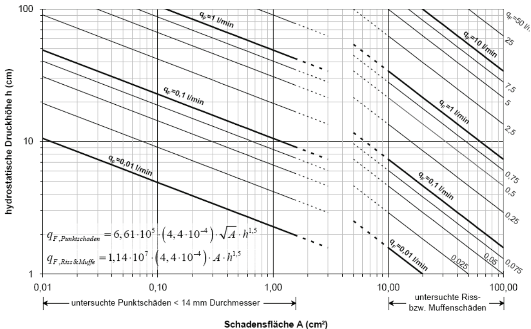
Abbildung 21: Grundwasserinfiltration q_F in Abhängigkeit der Schadensfläche und der hydrostatischen Druckhöhe für den rolligen Boden II (Hennerkes 2006)
