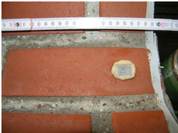
A: Abrieb im Randbereich des geklinkerten Gerinnes
